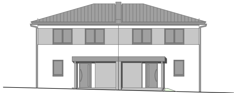
NORDANSICHT HAUS 2,4,6,8,10
